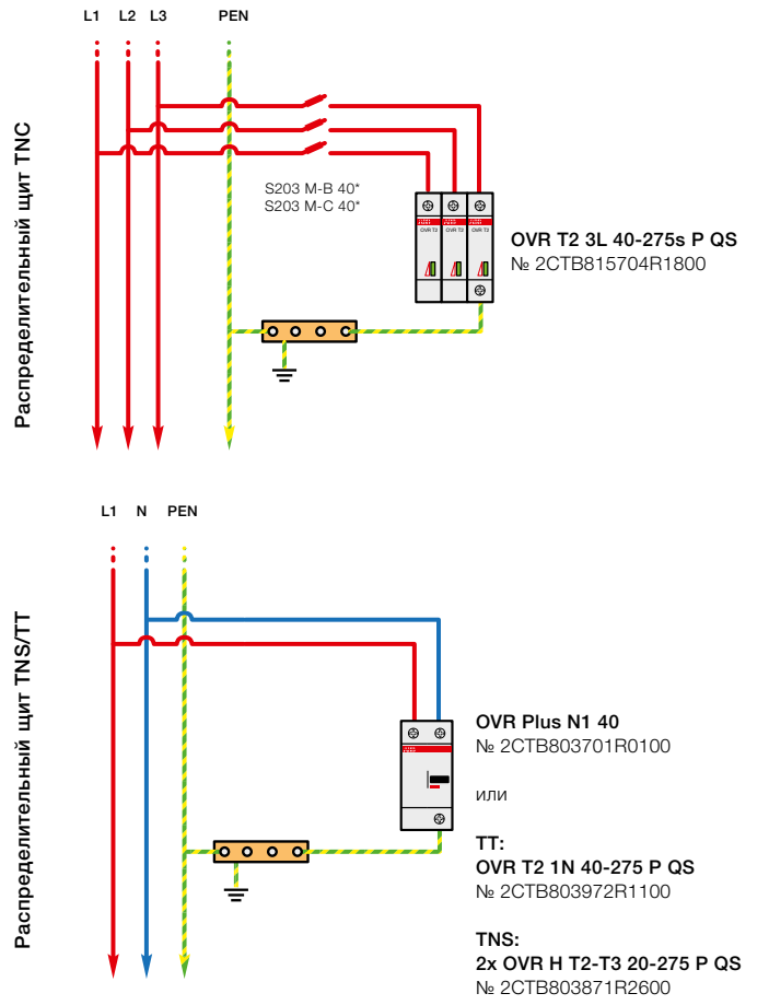
Конфигурация 2 С риском косвенных перенапряжений, переходных процессов
