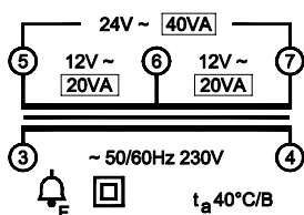
TM40/24
