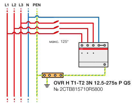
Конфигурация 3 I_p \leq 7 \text{ кА}
