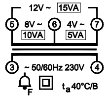
TM40/12
