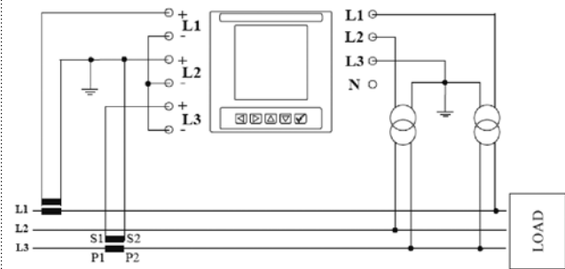
Подключение через 2 ТТ и 2 ТН (схема Арно)
