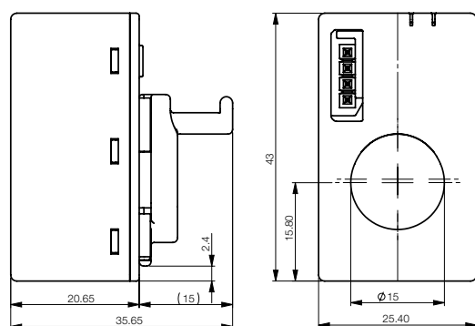
Датчик (CMS-200CA)
