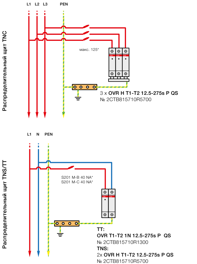
Конфигурация 1 С риском прямого попадания молнии (внешняя защита, воздуш. линии)
