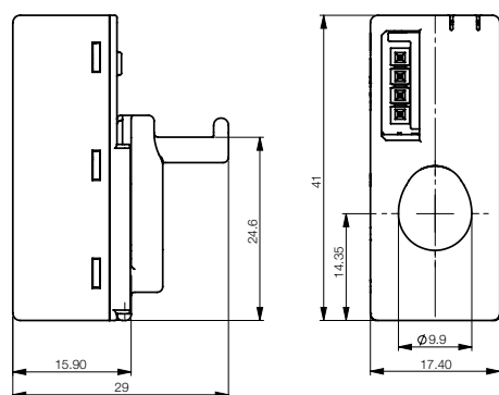
Датчик (CMS-100CA)
